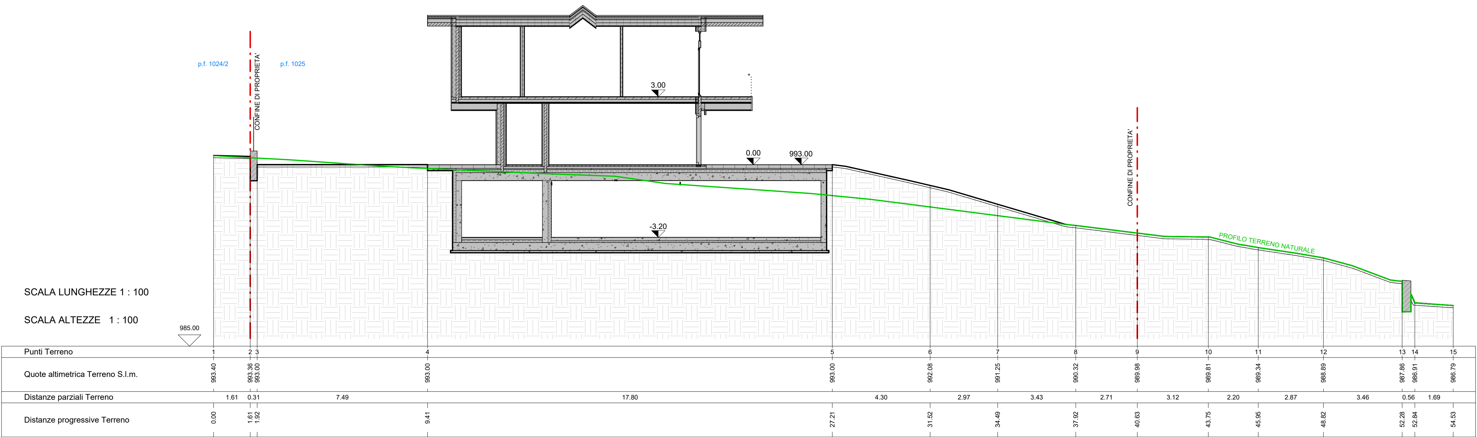
S.alt 1 SDP 1 : 100
