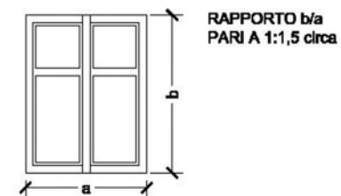
TELAIO CON PARTITURA QUATTRO SPECCHI (SPECCHI SUPERIORI QUADRATI)
